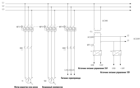
Сигловое схемо
