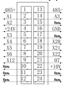
24 контактный распределитель
